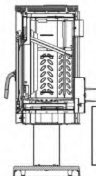
Schéma de principe : Vue en coupe du déflecteur
